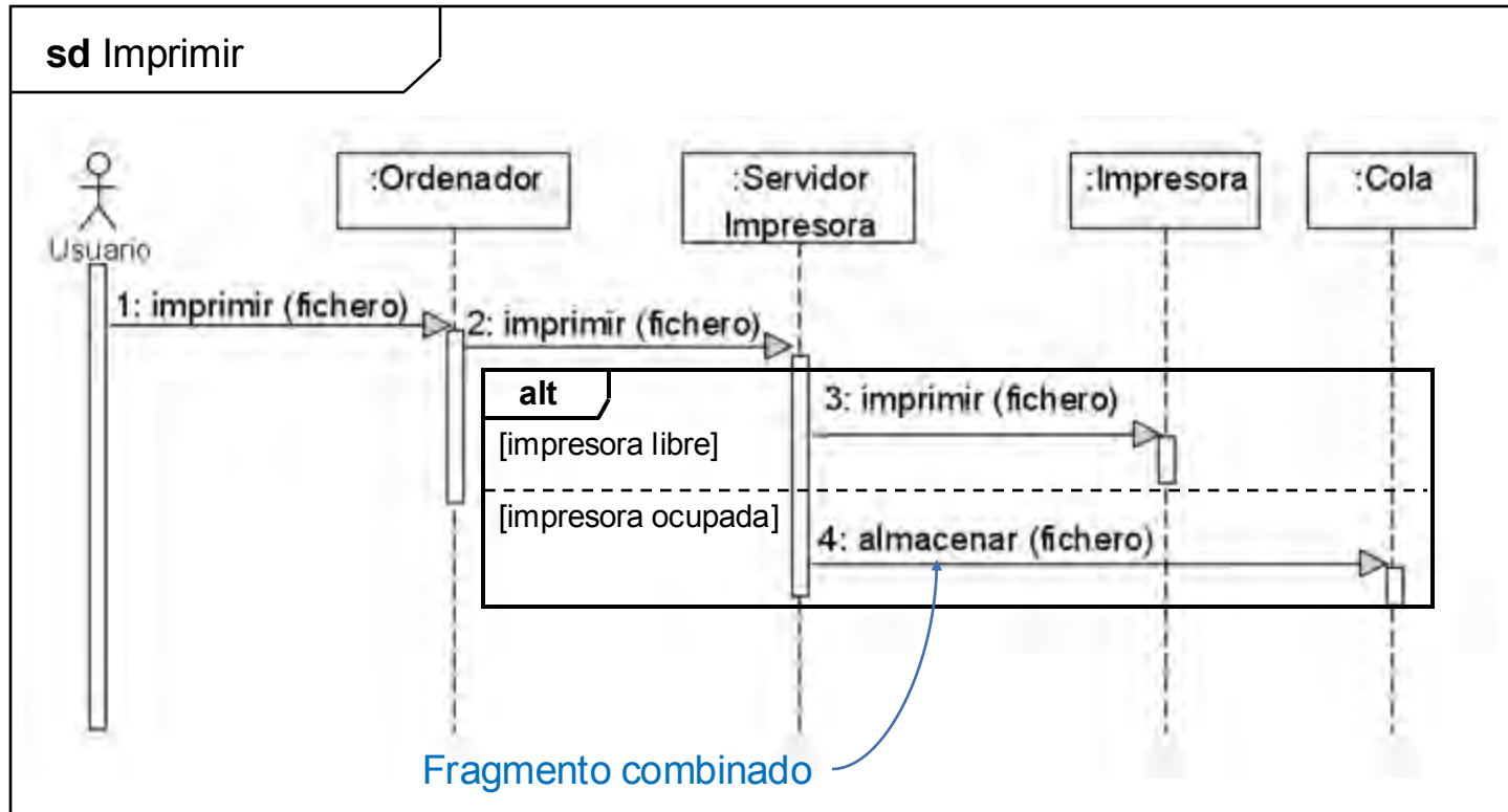
Diagrama de secuencia con un fragmento combinado
