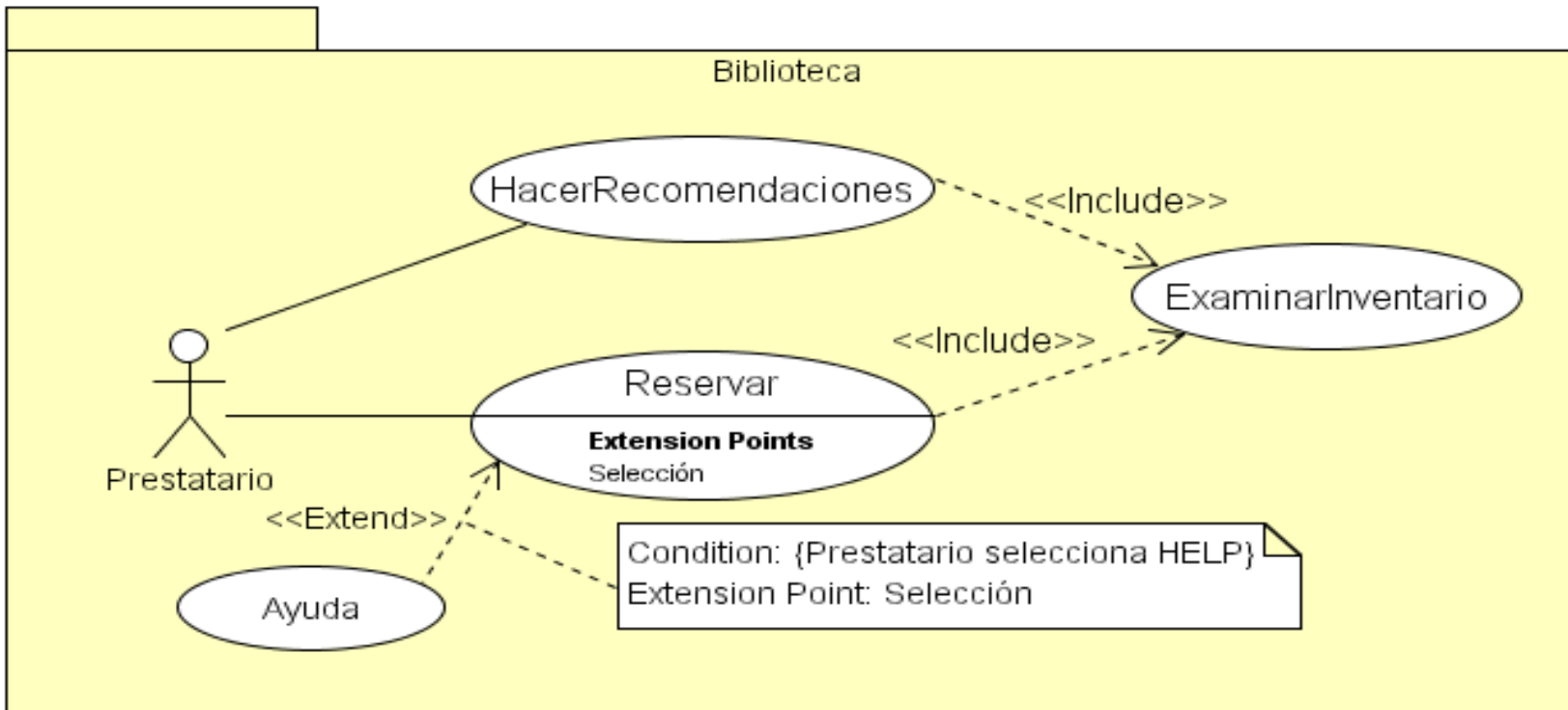
Diagrama de casos de uso del paquete Biblioteca
