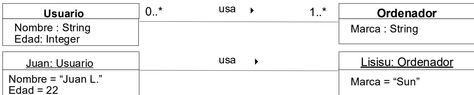
Diagrama de clases y diagrama de objetos
