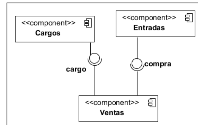
Diagrama de componentes
