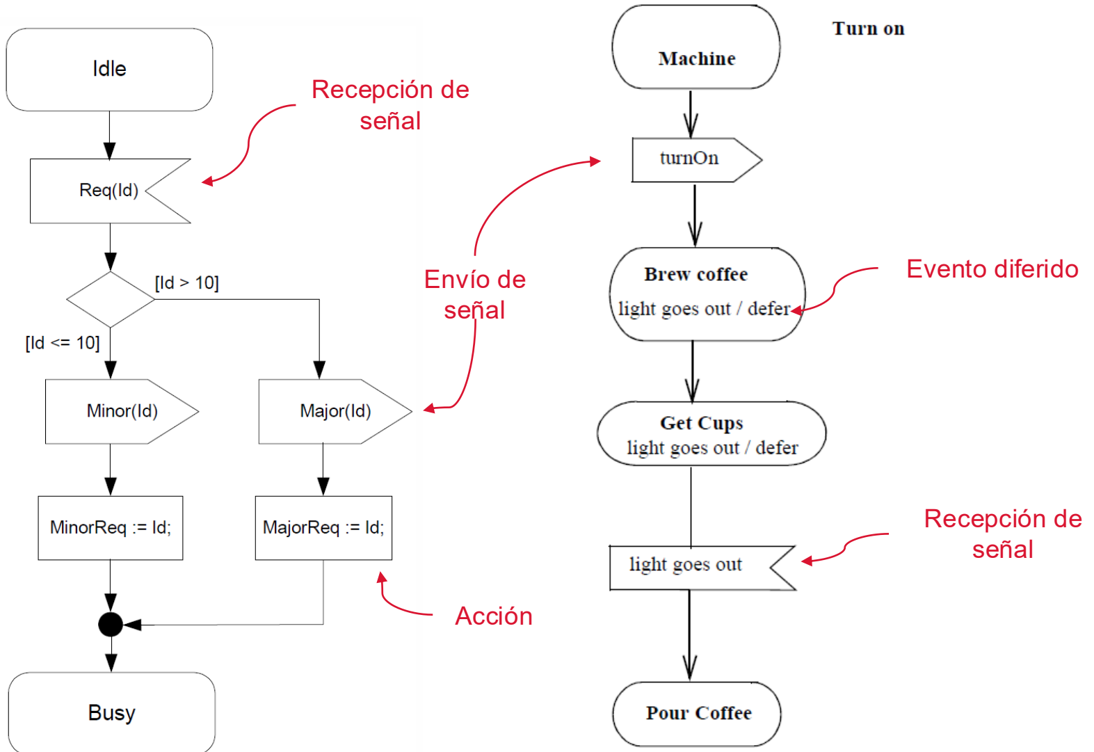
Ejemplos de representación de envío y recepción de señales y acciones en las transiciones
