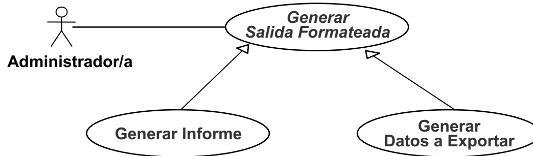
Relaciones de generalización entre casos de uso
