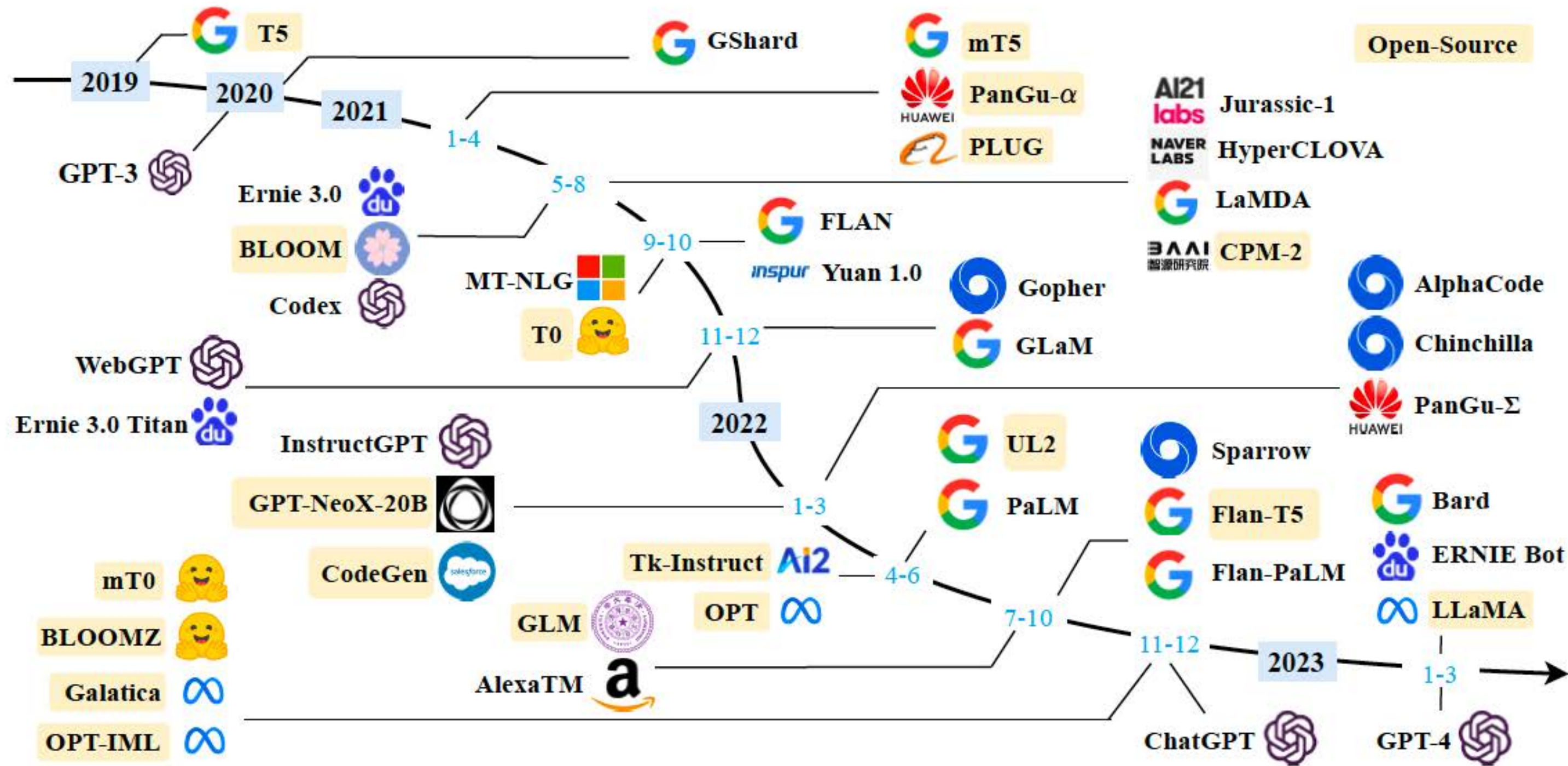
Cronología de los grandes modelos de lenguaje existentes (con un tamaño superior a 10.000 millones de parámetros) en los últimos años (en amarillo se marcan los LLM de código abierto). Fuente: [16]
